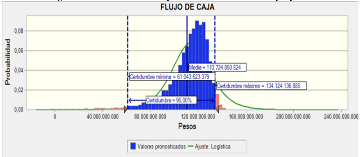
Figura 10-3 Distribución de probabilidad del VPN del proyecto
