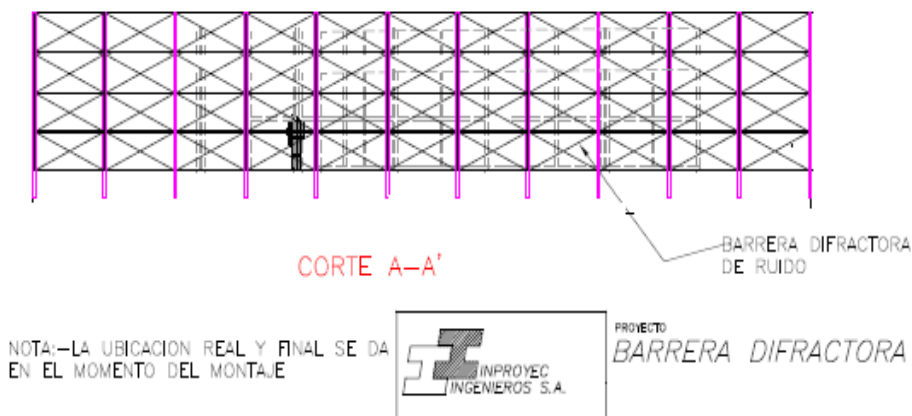
Figura 11-19 Esquema de una barrera difractora de ruido convencional
