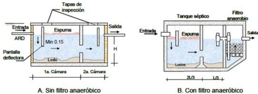
Figura 11-8 Esquema básico de un tanque séptico
