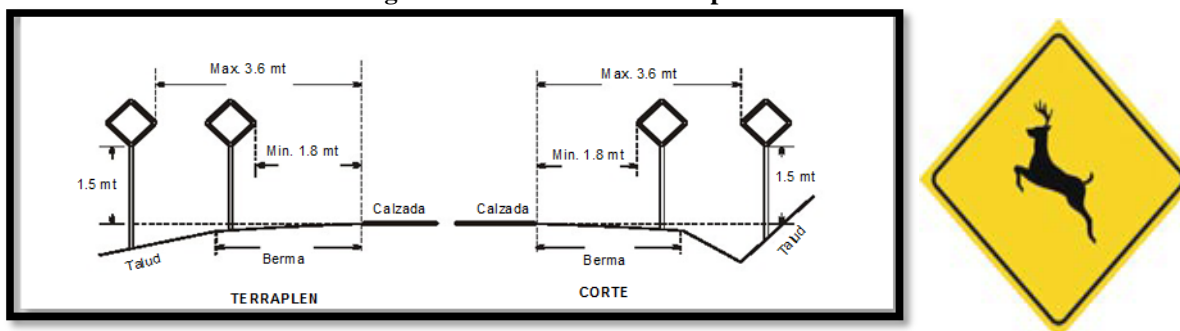
Figura 11-20 Señalización vial para fauna
