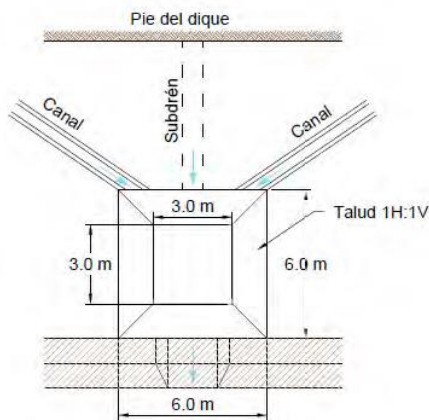
Figura 11-17 Esquema en planta de piscina desarenadora
