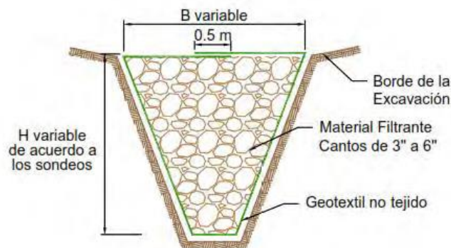
Figura 11-16 Filtro de subdrenaje típico
