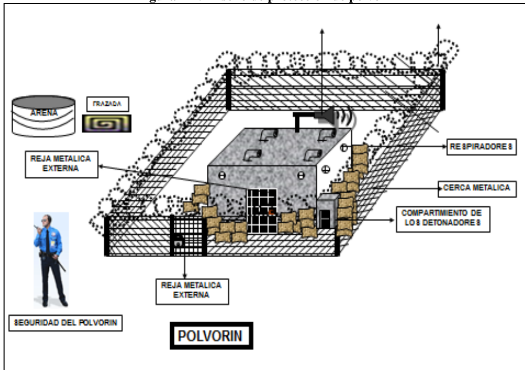
Figura 11-5 Diseño de protección de polvorín
