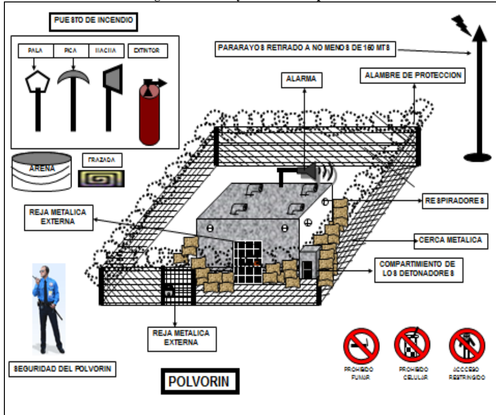
Figura 11-6 SST y señalización polvorín
