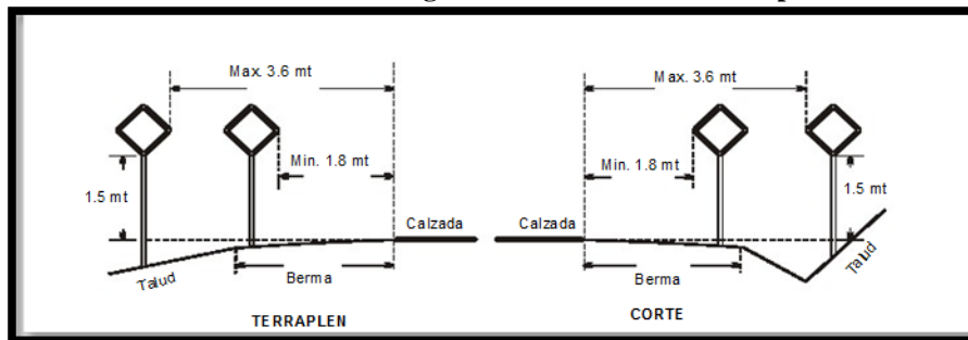
Figura 11-22 Señalización vial para fauna
